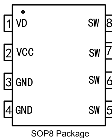
Fig.1. G3687CF Pin Configuration
